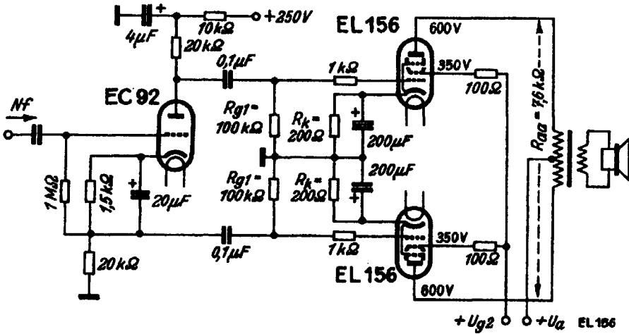
Prinzipschaltung für Gegentakt-AB-Betrieb mit Kathodenwiderständen und EC 92 als Phasenumkehröhre. Sprechleistung 80 Watt.
