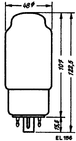
Kolbenabmessungen
