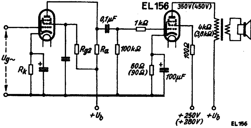
Prinzipschaltung für Eintakt-A-Betrieb mit Pentodenvorstufe. Sprechleistung 15 Watt. (Werte in Klammern gelten für eine Sprechleistung von 25 Watt.)
