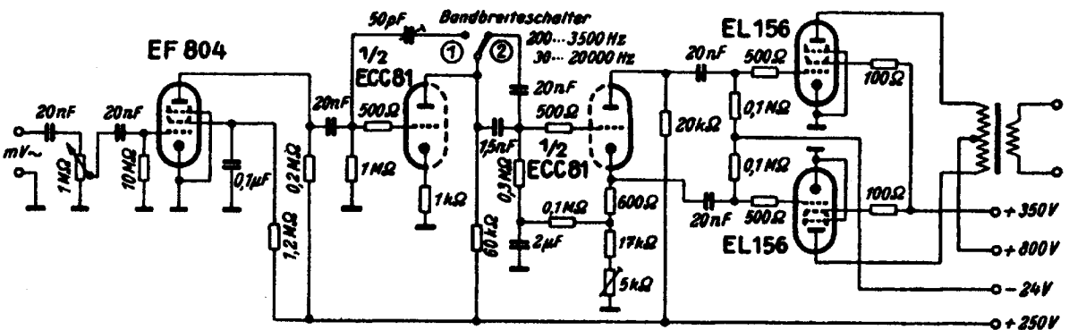
Modulationsverstärker für Amateursender (Nf-Leistung 120 W). Geignet für Anodenmodulation der Röhren EL 152 / EL 153
